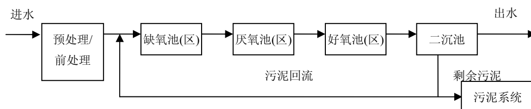
图 A.4 RAAO 工艺流程图
